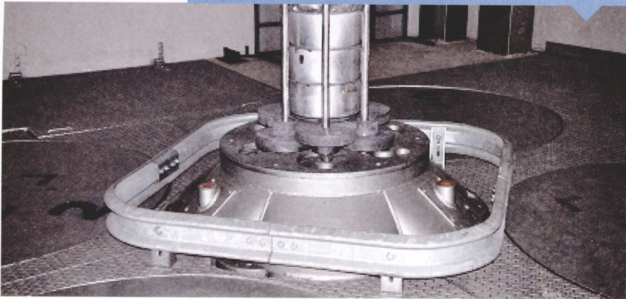
ตัวเครื่องฉายรังสีแกมมา ใช้ต้นกำเนิดรังสีโคบอลต์-60 จำนวนทั้งหมด 6 แท่ง ซึ่งแต่ละแท่งมีความแรงประมาณ 12,000 คูรี ความแรงรังสีรวมทั้งหมด 70,500 คูรี ปัจจุบันความแรงรังสีลดลงเหลือ 49,374 คูรี ผลิตโดยบริษัท Paul Stephens Consultancy Ltd. ประเทศอังกฤษ
