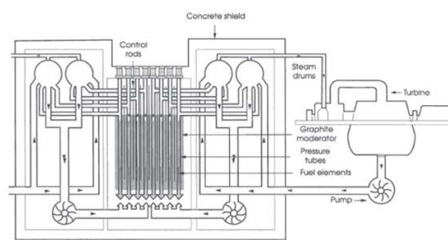
โรงไฟฟ้านิวเคลียร์แบบ RBMK
