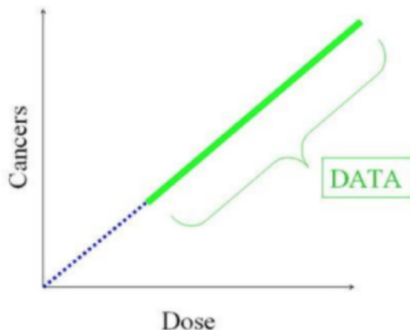
รูปที่ 1 การทำนายอุบัติการณ์การเกิดมะเร็งจากการได้รับรังสี โดยใช้วิธีนำข้อมูลผลของรังสีจากการได้รับปริมาณสูง ๆ (จากการใช้ระเบิดปรมาณูในสงครามโลกครั้งที่ 2 อุบัติเหตุทางนิวเคลียร์ การรักษาผู้ป่วยมะเร็งซึ่งได้รับรังสีสูงเฉพาะที่) และลากเส้นต่อลงมาเพื่อทำนายผลของรังสีปริมาณต่ำ ๆ (รูปจาก Brooks AL. Defining Low-Dose Cancer Risks. 8 Aug 2007. www.tricity.wsu.edu/faculty/brooks/LasVegas1.ppt )
