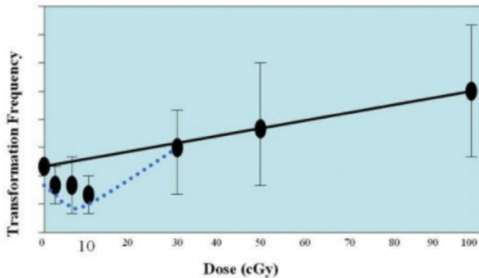
รูปที่ 2 ปริมาณรังสีต่ำ ๆ ทำให้การเปลี่ยนแปลงของโครโมโซมลดลง (รูปจาก Brooks AL. Defining Low-Dose Cancer Risks. 8 Aug 2007. www.tricity.gov.au/faculty/brooks/LowDoseCancer1.pdf )
